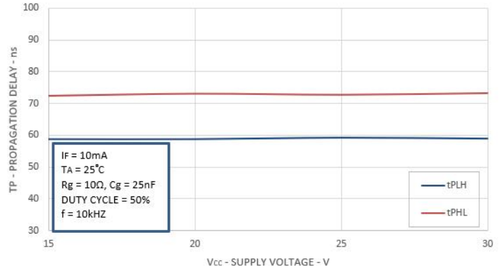
图例 8-传输延时与电源电压曲线图
