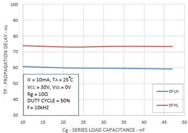
图例 12-传输延时与电容曲线图
